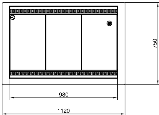
Planta
